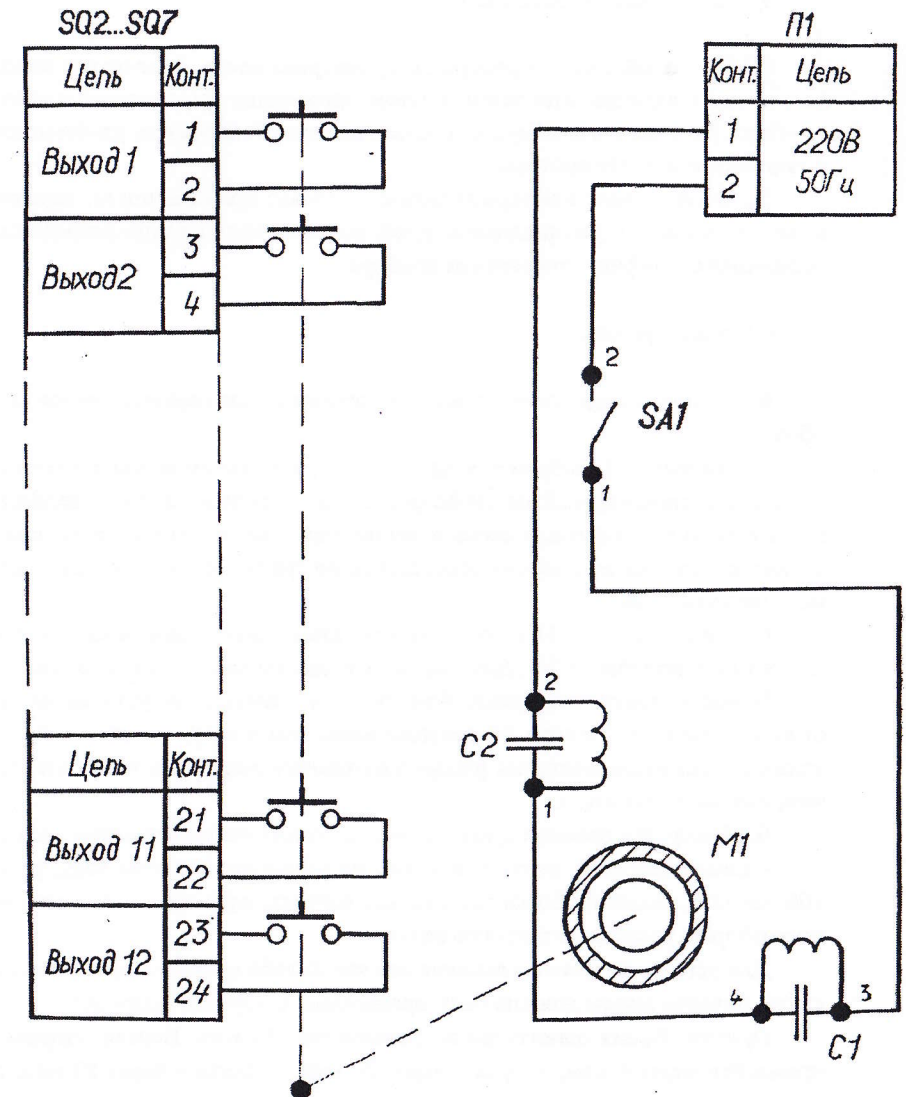
П1 – панель питания; SA1 – тумблер TB2-1; SQ2 – SQ7 – контактная группа; M1 – электродвигатель СД-54 (1/137); C1 – конденсатор МБГЧ-1-2А-250-0,5±10%; C2 – конденсатор МБГЧ-1-2А-250-2,0±10%.
