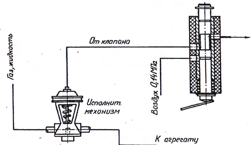
II. Положение поршня золотника при сброшенной защелке выключателя КЭП-12У
