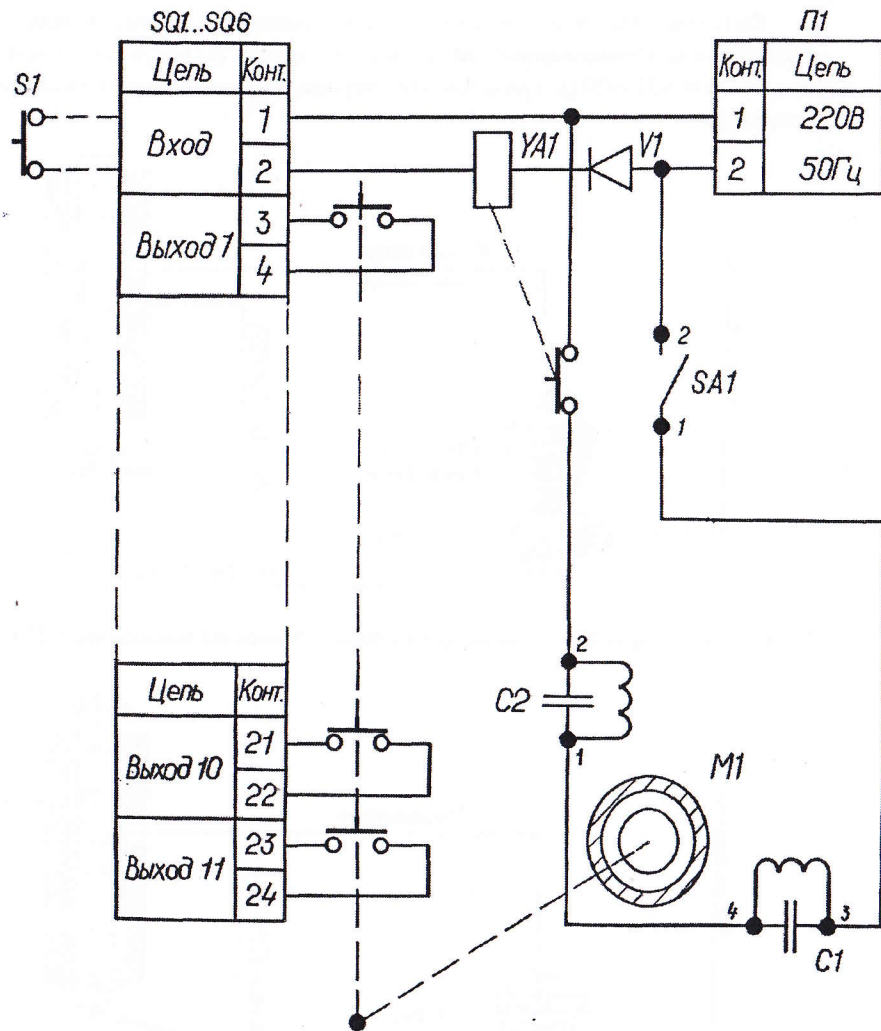
П1 – панель питания; SA1 – тумблер TB2-1; S1 – выключатель; YA1 – электромагнит; SQ1 – SQ6 – контактная группа; M1 – электродвигатель СД-54 (1/137); C1 – конденсатор МБГЧ-1-2А-250-0,5±10%; C2 – конденсатор МБГЧ-1-2А-250-2,0±10%; V1 – диод Д226Б.
