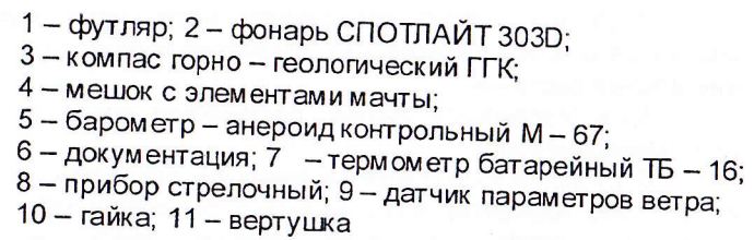
Рисунок 1 – Метеокомплект уложенный в футляр
